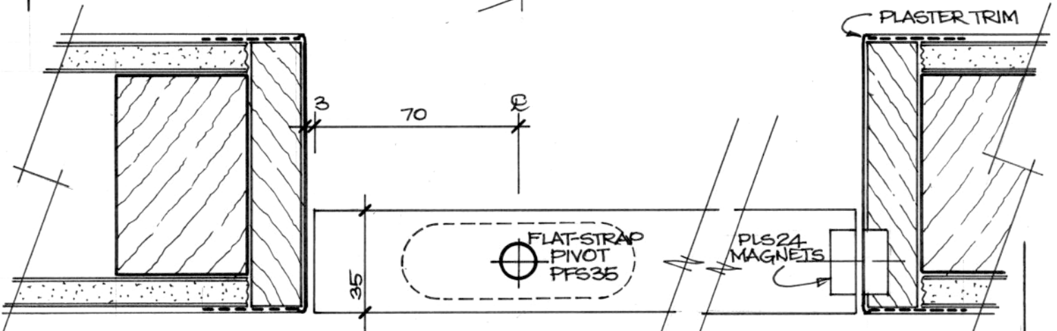
PIVOT JAMB
