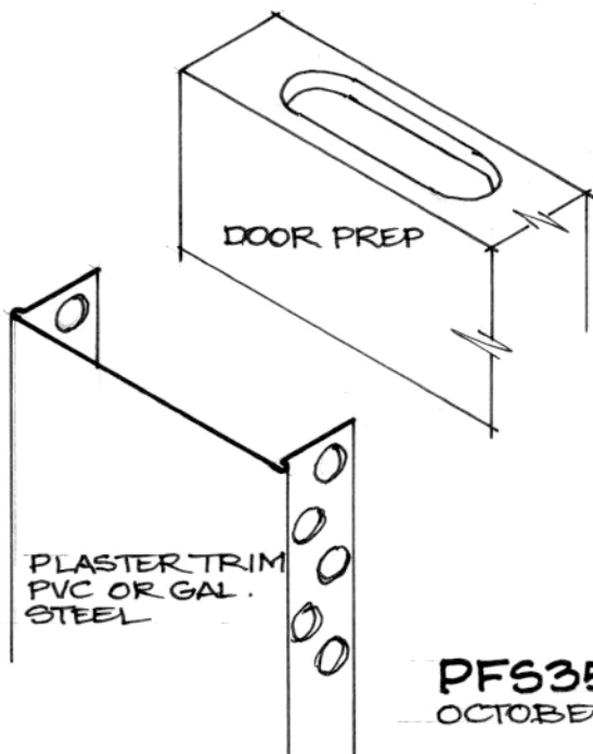
PIVOT JAMB
